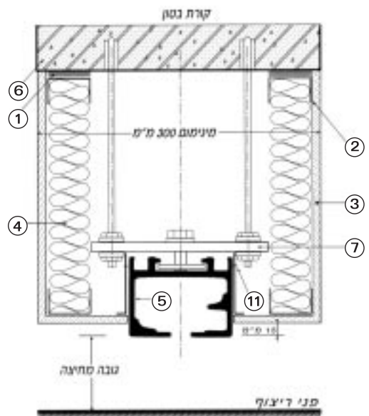
ג. פרט חיפוי מערכת התליה עם קורת בטון
