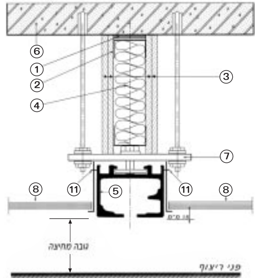
א. התחברות של תקרה אקוסטית למסילת המחיצה
