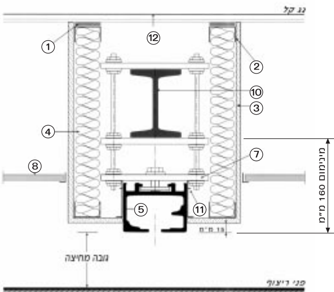
ד. פרט חיפוי קורת פלדה ומערכת התליה
