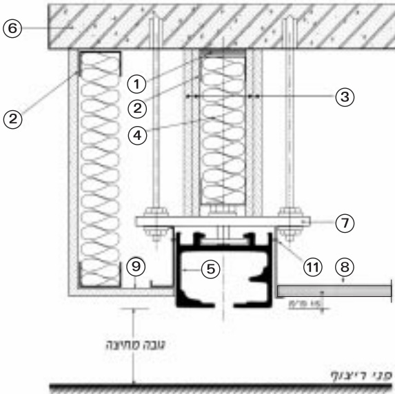
ב. התחברות של תקרה אקוסטית/גבס או קרניז למסילת המחיצה
